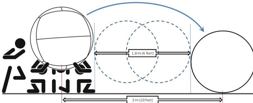
Figure 5 : Distance minimale que le ballon doit parcourir.
